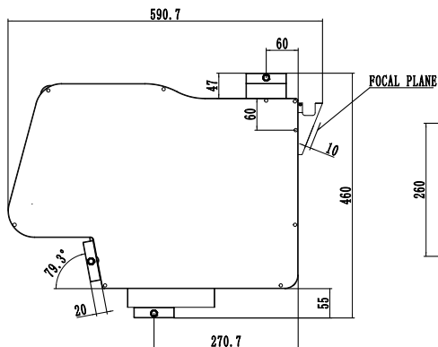
光谱仪HiperS-3208i外形尺寸图
