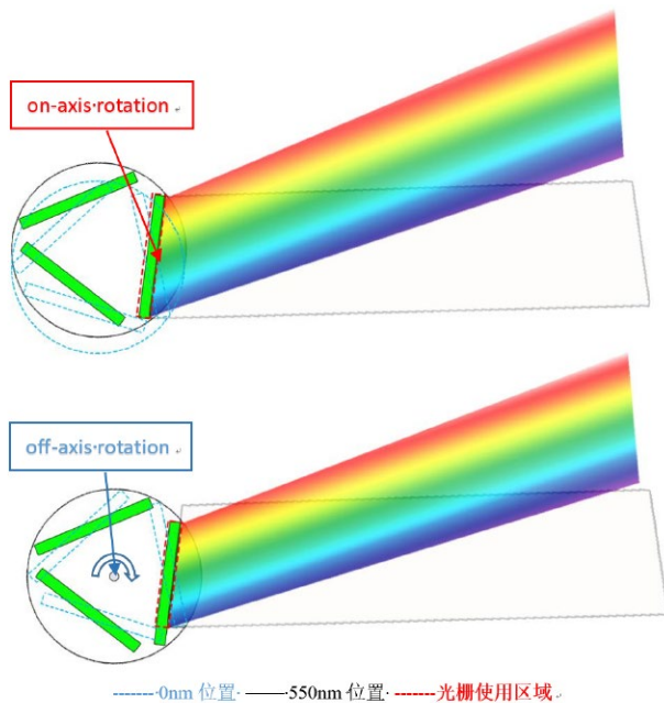
光栅在轴旋转光栅利用率提高 15%。（1200g/mm 光栅，波长 550nm 位置）
